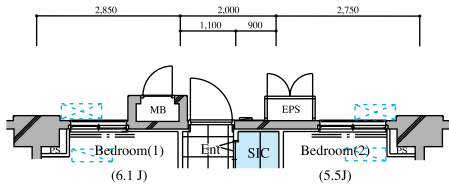
621、719、820号室部分図
