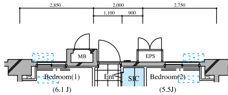
623、721、822号室部分図
